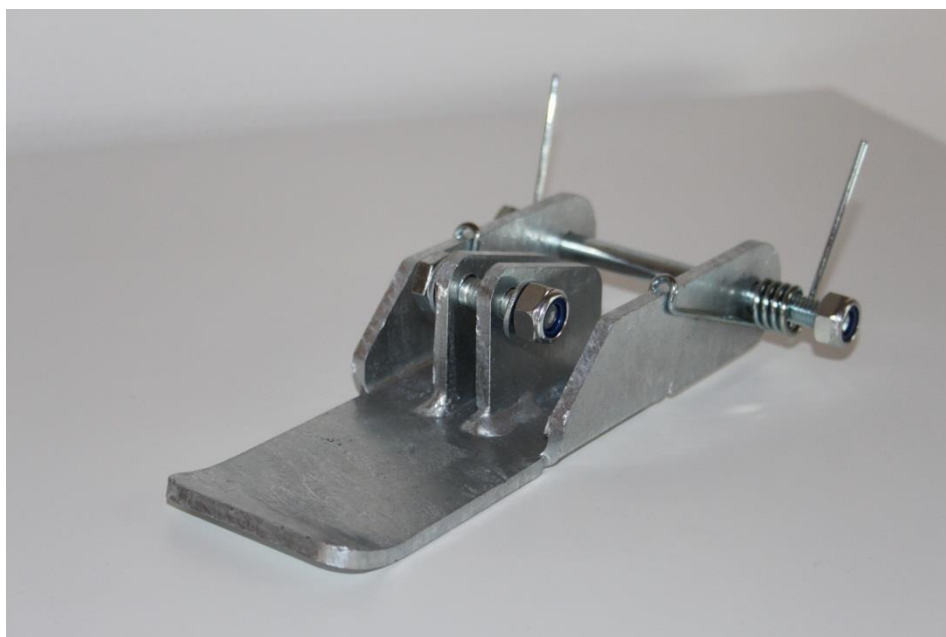
VARE NR. 1946 FOD TIL AFRULNINGSSIKRING KOMPLET
